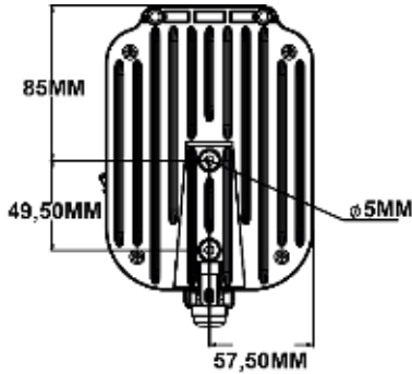
Şekil 8 Nano Seri Pompa Ebatı Arka Kısım
