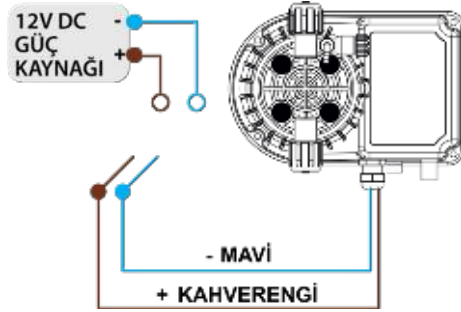
Şekil 13 DC Modeller İçin Elektrik Bağlantısı
