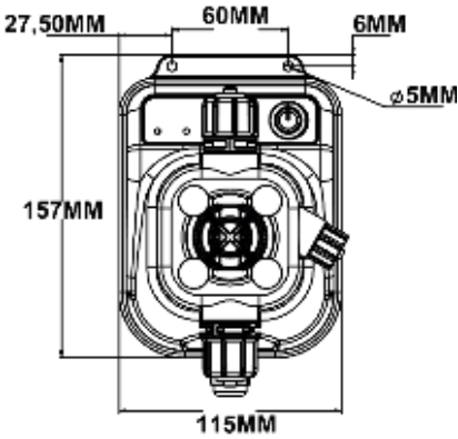
Şekil 5 Nano Seri Pompa Ebatı Ön Kısım
