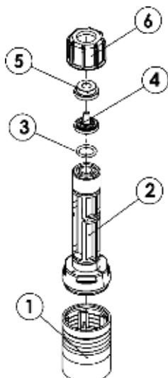
Şekil 21 Emiř Hattı Montaj Sıralaması
