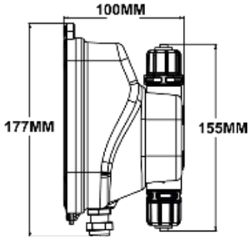
Şekil 7 Nano Seri Pompa Ebatı Yan Kısım
