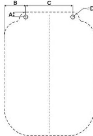
Şekil 9 Nano Seri Pompa Montaj Delik Ölçüleri
