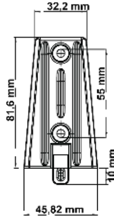
Şekil 6 Nano Seri Pompa Askı Aparatı Ebatı
