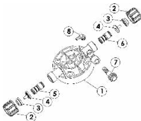
Şekil 22 Kafa Takımı 40-50 Montaj Sıralaması
